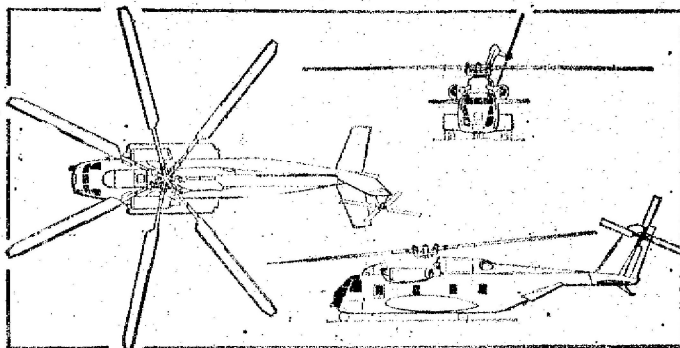
53 סיקורסקי — כלליות המסוק
